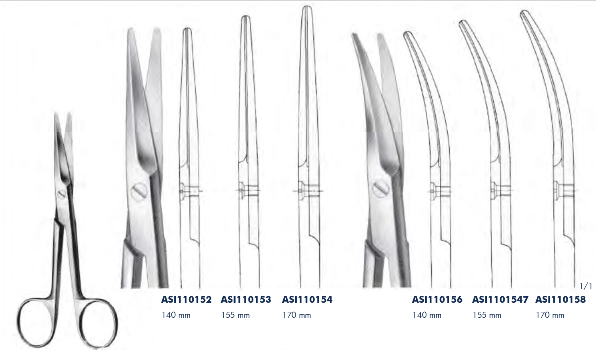
TUBBS ASI110152 - ASI110158
