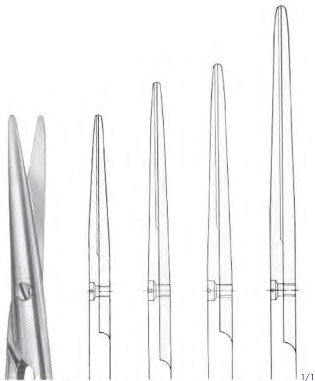
ASI110201 230 mm ASI110202 250 mm ASI110203 280 mm ASI110204 305 mm
