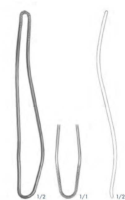
FRENZEL ASI250772 165 mm
