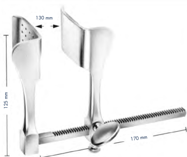
TUFFIER ASI200541 Blades 43 x 53 mm
