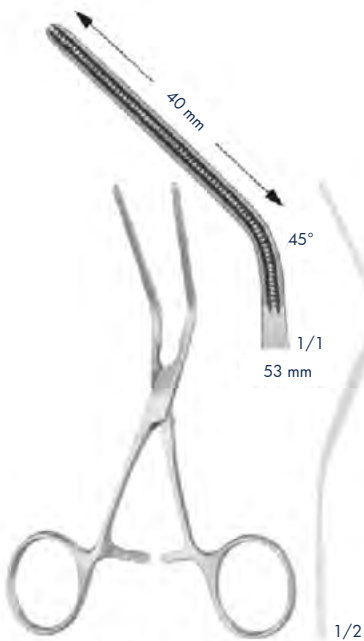
DE BAKAY ASI200243 angled 45° 125 mm
