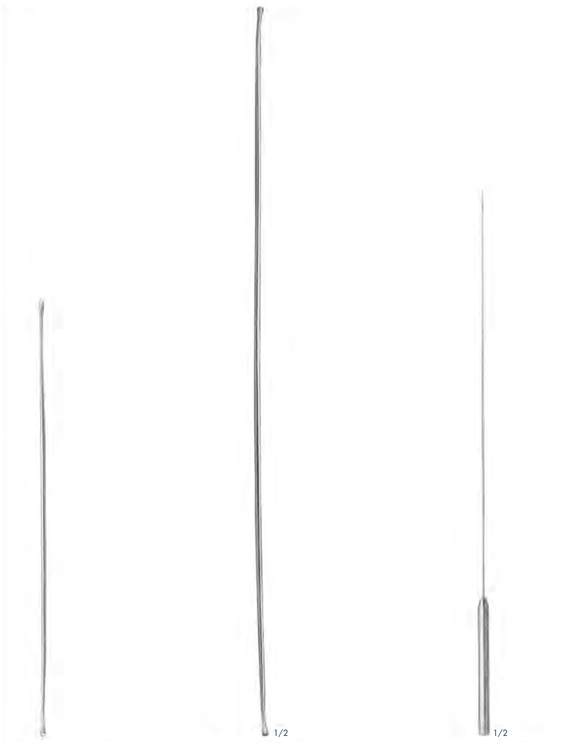
Ø Tip ASI160233 1,5 mm ASI160234 2,0 mm ASI160235 2,5 mm Probes 300 mm
